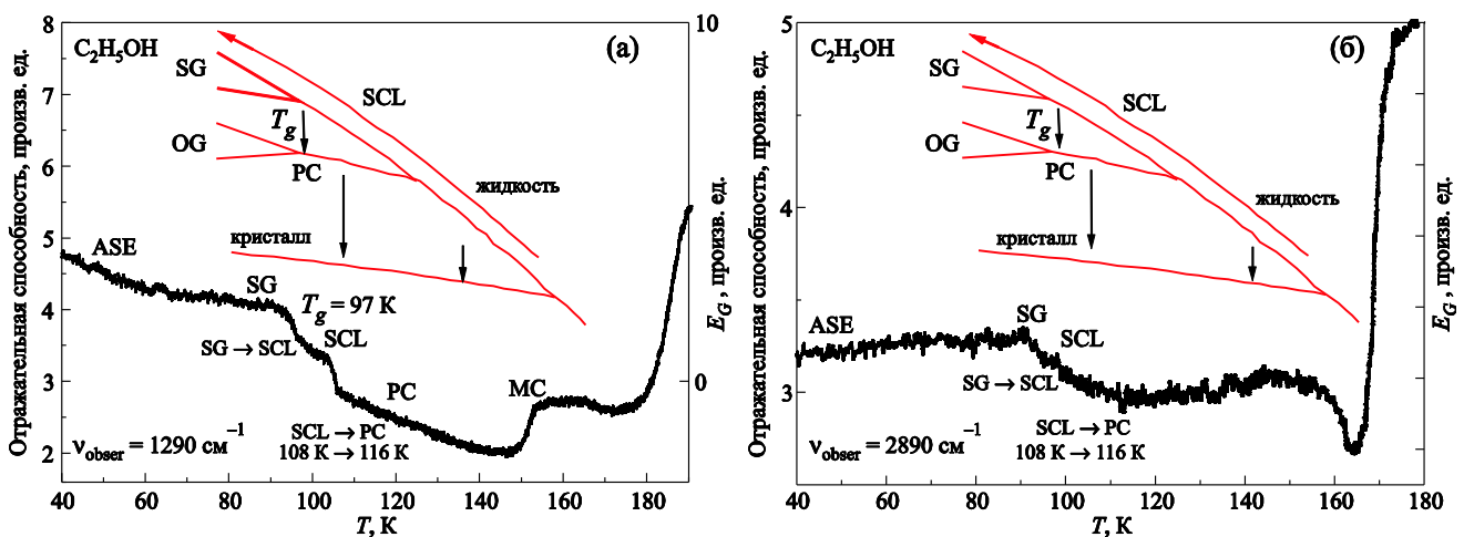
Рис. 2. Изменение сигнала ИК спектрометра на частоте наблюдения \nu = 1290 \text{см}^{-1} (а) и \nu = 2890 \text{см}^{-1} (б) при повышении температуры пленки этанола. T_c = 16 К, d = 1,5 нм, давление конденсации P = 5 \cdot 10^{-5} Торр.
