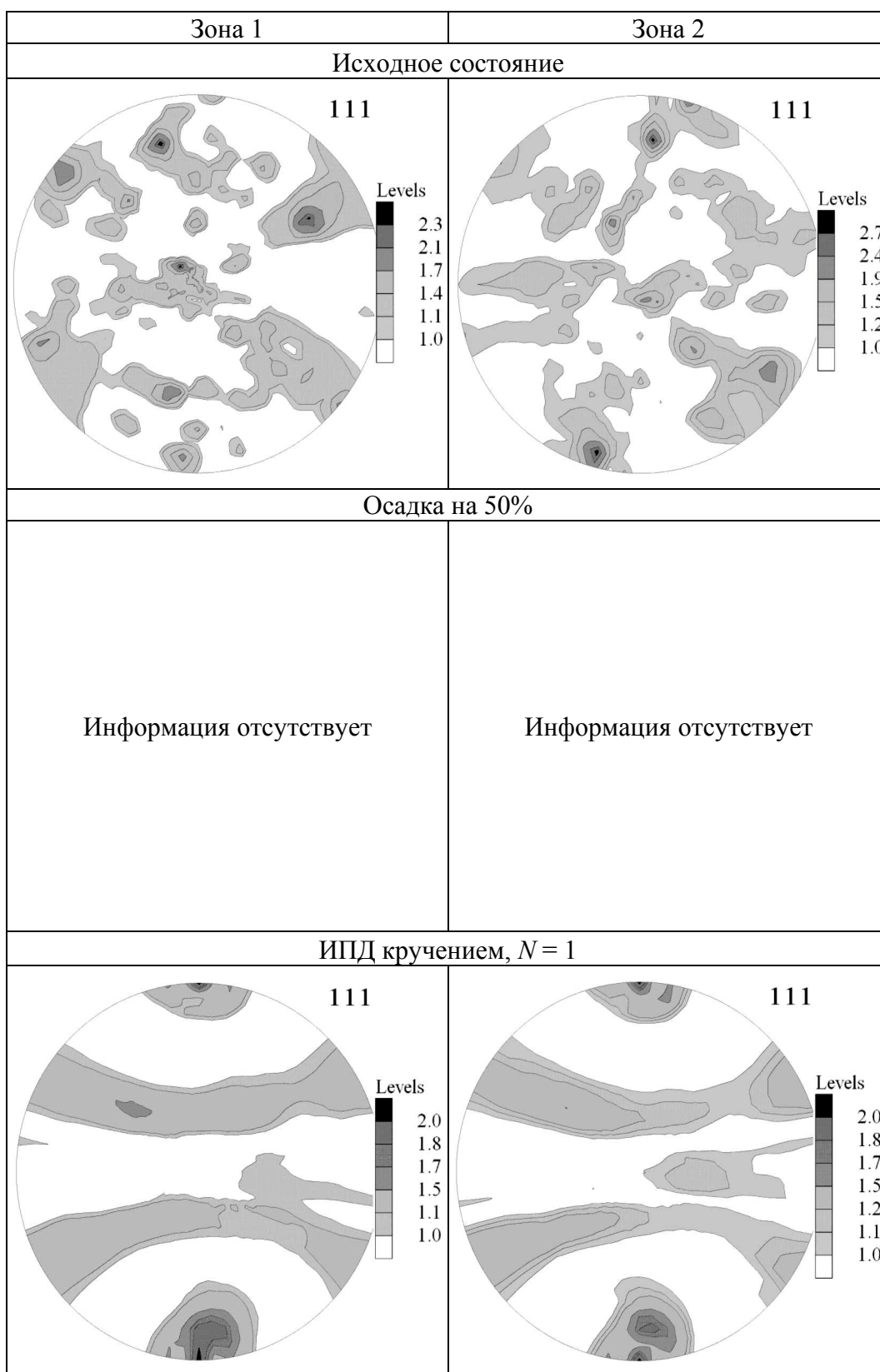
Рис. 2. Экспериментальные ПФ (111)
