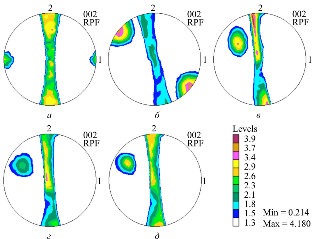
Рис. 2. Экспериментальные ПФ (0002) для Ti Grade 4 в различных состояниях: a – исходной, б – 1 проход РКУП-К, в – 2, г – 4, д – 8 проходов. Продольное сечение, T = 400^{\circ}\text{C}
