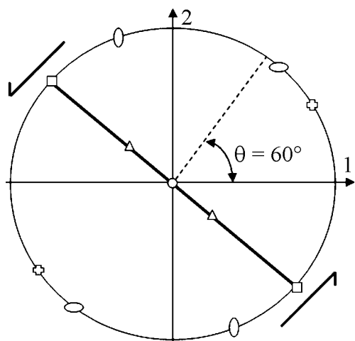
Рис. 3. Положения идеальных ориентировок простого сдвига при РКУП-К на ПФ (0001) для металлов с ГПУ-решеткой ( c/a = 1.633 ) [12]: \square – H1_{\theta} , \circ – H2_{\theta} , \Delta – H3_{\theta} , \oplus – H4_{\theta} , \diamond – H5_{\theta} , \circ – H6_{\theta} . Угол пересечения каналов 120^{\circ}
