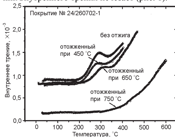
Рис. 1. Зависимость внутреннего трения от температуры отжига для покрытия типа nc\text{-TiN}/\alpha\text{-Si}_3\text{N}_4 , полученного магнетронным распылением [13].
