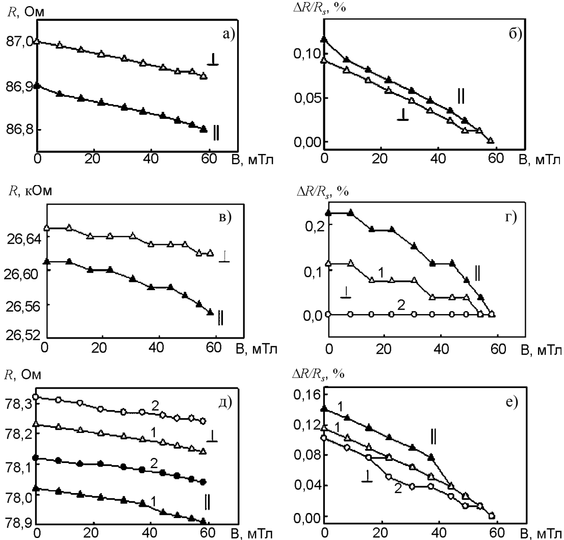
Рис. 2. Залежність R(B) і \frac{\Delta R}{R_s}(B) для відпалених до T_c \cong 850 К плівок Pd(3) (а, б), Fe(3) (в, г) та Pd(3)/Fe(3)/Π (д, е) із ГЦТ решіткою. В дужках вказана товщина в нм. 1, 2 – номери циклів намагнічування.
