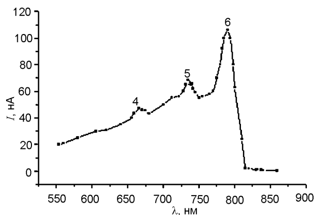
Рис. 3. Спектральное распределение фоточувствительности барьера Шоттки Al-pCdTe в длинноволновой области спектра.
