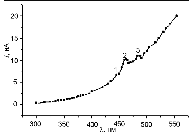
Рис. 2. Спектральное распределение фоточувствительности барьера Шоттки Al- pCdTe в коротковолновой области спектра.
