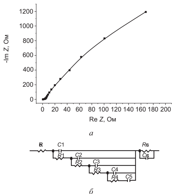
Рис. 2. Діаграма Найквіста (а) усіх досліджених матеріалів та відповідна електрична схема (б)
