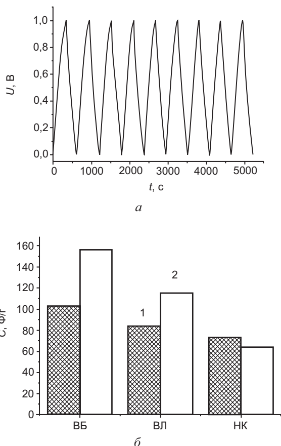
Рис. 1. Гальваностатичні цикли «заряд-розряд» (а) та питома ємність (б) межі розділу 30 % водного розчину КОН з вихідними (1) та обробленими ультразвуком (2) матеріалами
