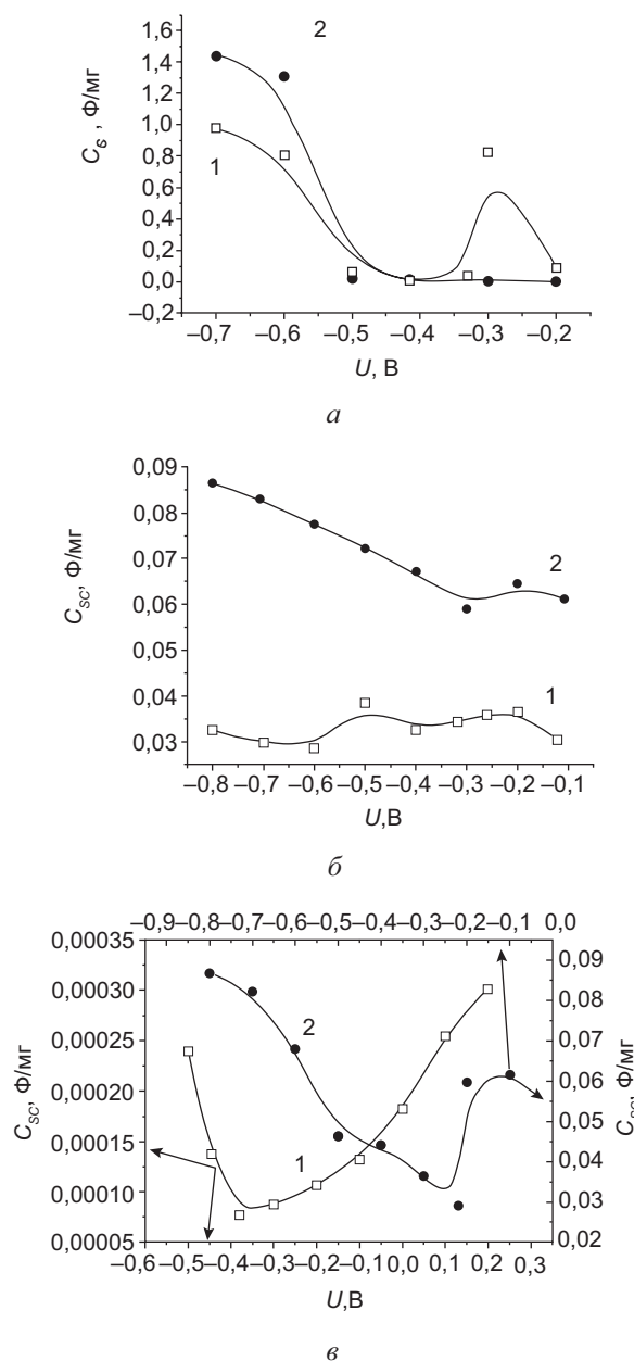
Рис. 3. Вольт-фарадні залежності для НК (а), ВБ (б), ВЛ (в) до (1) та після (2) ультразвукової обробки
