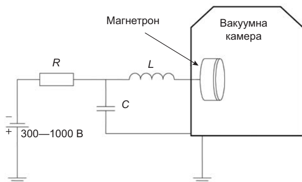
Рис. 3. Схема пасивного захисту від утворення мікродуг
