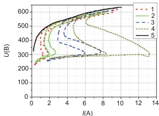
Рис. 9. ВАХ магнетронного розряду в аргоні з киснем, мішень з алюмінію. Тиск аргону p = 1,5 \cdot 10^{-3} Тор, газопотік кисню q : 1 — q = 5,5 см 3 /хв; 2 — q = 7,5 см 3 /в; 3 — q = 13,5 см 3 /хв; 4 — q = 21,5 см 3 /хв; 5 — q = 0 см 3 /хв
