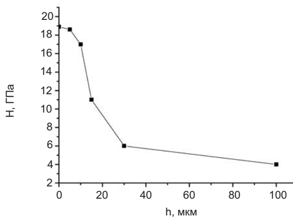
Рис. 5. Зависимость изменения твердости (Н) по глубине (h) после азотирования стали 12X18H10T с покрытием из Мо
