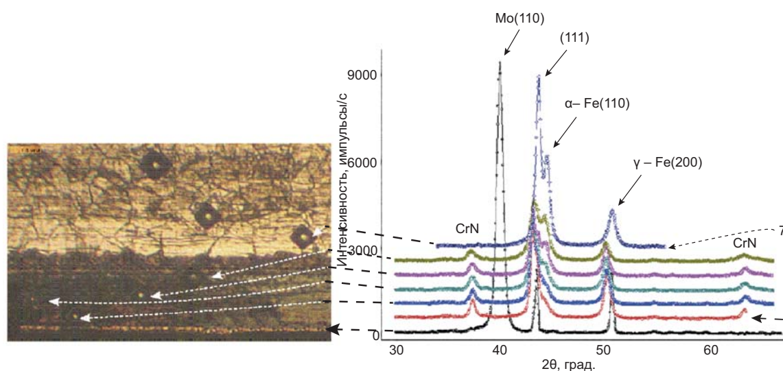
Рис. 7. Послойный анализ стали после азотирования (микрофотография шлифа боковой поверхности с отпечатками испытаний твердости и участки рентгендифракционных спектров): 1 — с покрытием Мо. После азотирования: 2 — с поверхности, 3 — после сошлифовки 5 мкм, 4 — 10 мкм, 5 — 15 мкм, 6 — 30 мкм и 7 — 100 мкм)
