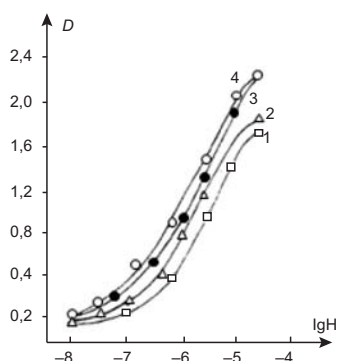
Рис. 11. Характеристические кривых фото процесса, измеренные для различных значений давления газа в зазоре. p , мм рт. ст.: 1 — 228; 2 — 138; 3 — 76; 4 — 38 U = 1,3 кВ, d = 60 мкм
