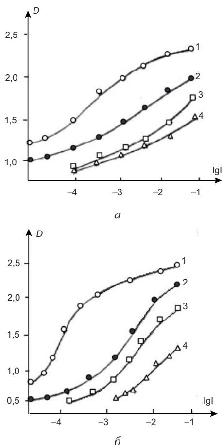
Рис. 9. Зависимости плотности почернения от интенсивности света при различных временах экспонирования 1 — 5 \cdot 10^{-4} с, 2 — 10^{-4} с, 3 — 5 \cdot 10^{-5} с, 4 — 2 \cdot 10^{-5} с полученные для арсенид галлиевого ФП прозрачного электрода (а) и при использовании светопровода с люминесцентным экраном (б). p = 76 мм рт. ст., d = 50 мкм, U = 1,8 кВ
