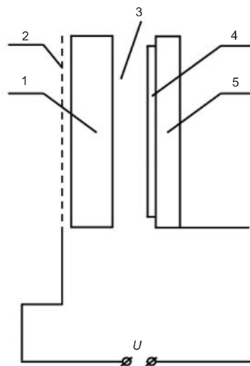
Рис. 1. Принципиальная схема полупроводниковой фотографической системы ионизационного типа
