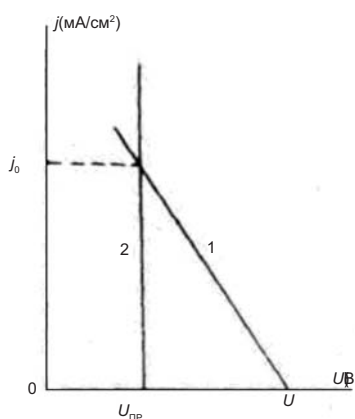
Рис. 7. График, поясняющий процесс управления током разрядного промежутка
