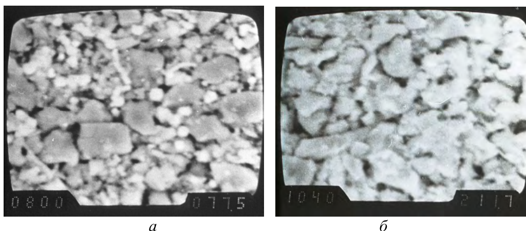
Рис. 1. Поведение частиц карбида титана и никеля (темное ограненное – TiC; светлое – Ni), \times 1000
