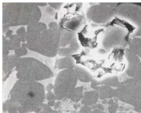
Рис. 6. Скопление карбидных частиц, \times 1000 и в 1,5 раза при печати, поляроид
