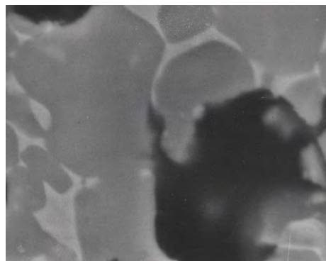
Рис. 7. Формирование арочной поры из карбидных частиц, \times 5000 и в 2 раза при печати, поляроид
