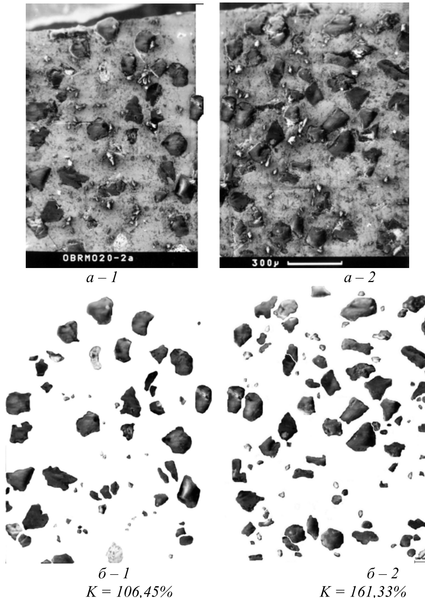
Рис. 4. Фотографии шлифа сегментов 1 и 2 режущего слоя экспериментального круга исходные (а – 1, а – 2) и откорректированные (б – 1, б – 2)
