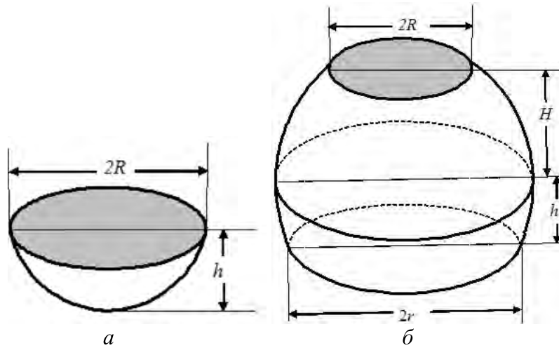
Рис. 3. Возможные варианты невидимой части среза зерна: а – шаровой сегмент, б – шаровой пояс
