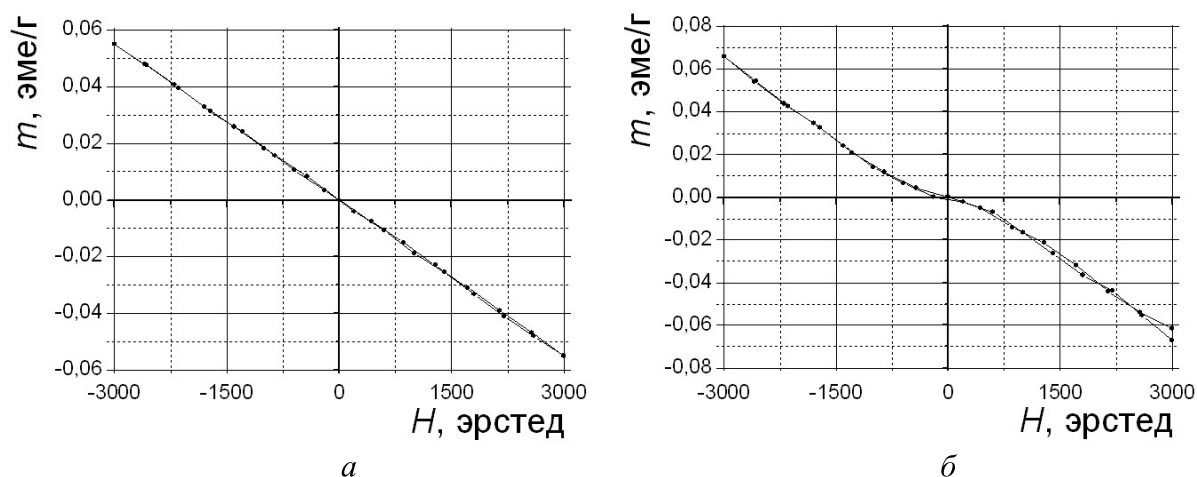
Рис. 1. Показания вибрационного магнитометра для образца: а – 1; б – 2
