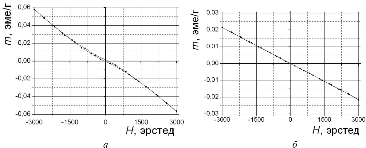
Рис. 3. Показания вибрационного магнитометра для образца: а – 3; б 4
