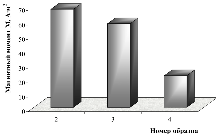
Рис. 4. Значения магнитного момента для образцов 2–4
