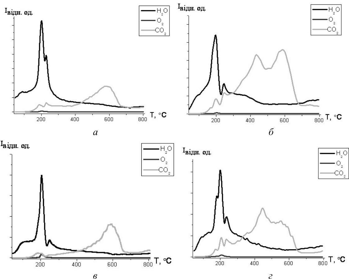
Рис. 3. Термодесорбционные спектры \text{H}_2\text{O} , \text{O}_2 и \text{CO}_2 с поверхности образца: ДНА (а) и АСУД-95 (б), модифицированного \text{CuO}\cdot\text{Fe}_2\text{O}_3 , ДНА (в) и АСУД-95 (г), модифицированного \text{CuO}\cdot\text{Co}_3\text{O}_4
