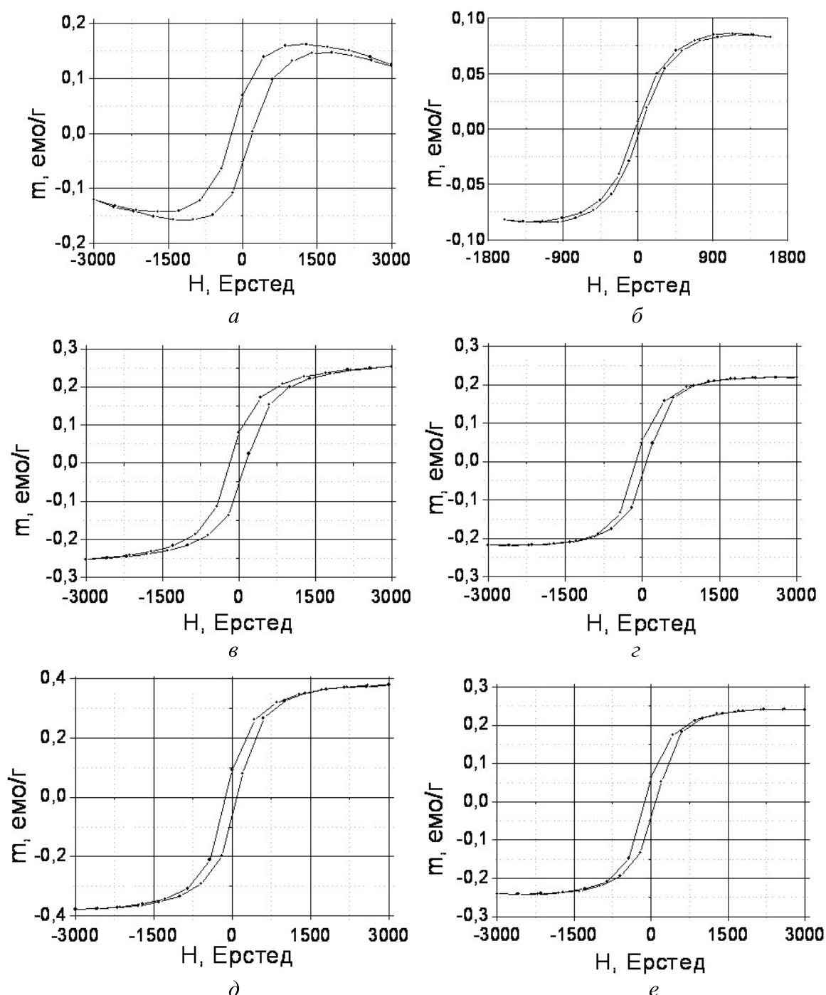
Рис. 4. Зависимость удельного магнитного момента образца наноалмаза от напряжённости магнитного поля (петля гистерезиса): ДНА (а) и АСУД-95 (б), ДНА (в) и АСУД-95 (г), модифицированного \text{CuO}\cdot\text{Fe}_2\text{O}_3 , ДНА (д) и АСУД-95 (е), модифицированного \text{CuO}\cdot\text{Co}_3\text{O}_4
