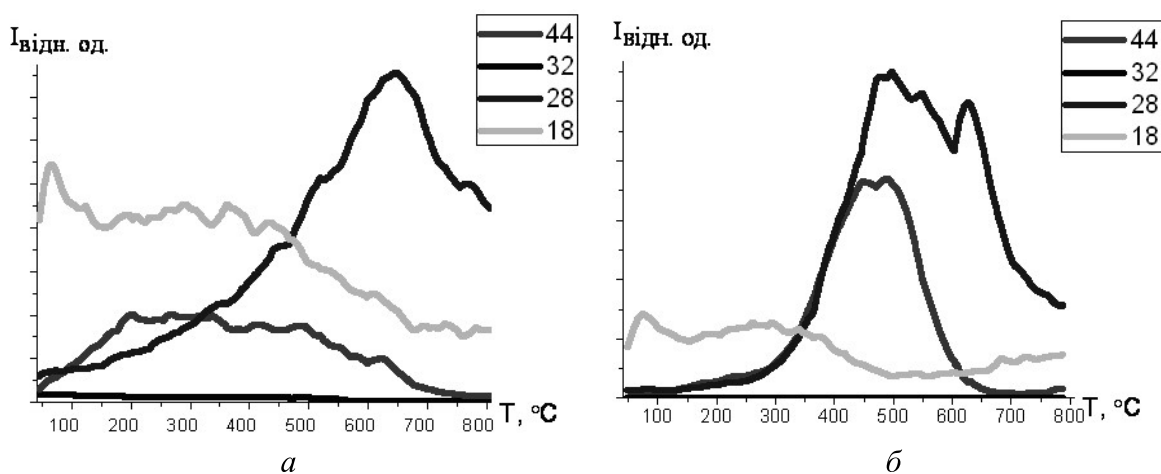
Рис. 2. Термодесорбционные спектры \text{H}_2\text{O} , \text{CO} , \text{O}_2 и \text{CO}_2 с поверхности образца: ДНА (а) и АСУД-95 (б)
