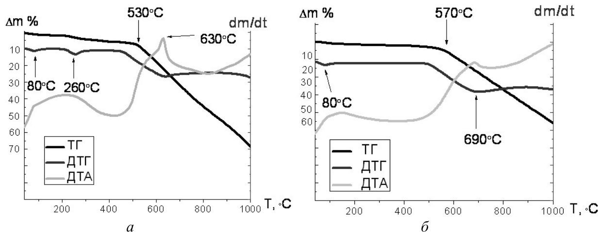
Рис. 1. Дериватограммы: ДНА (а) и АСУД-95 (б)
