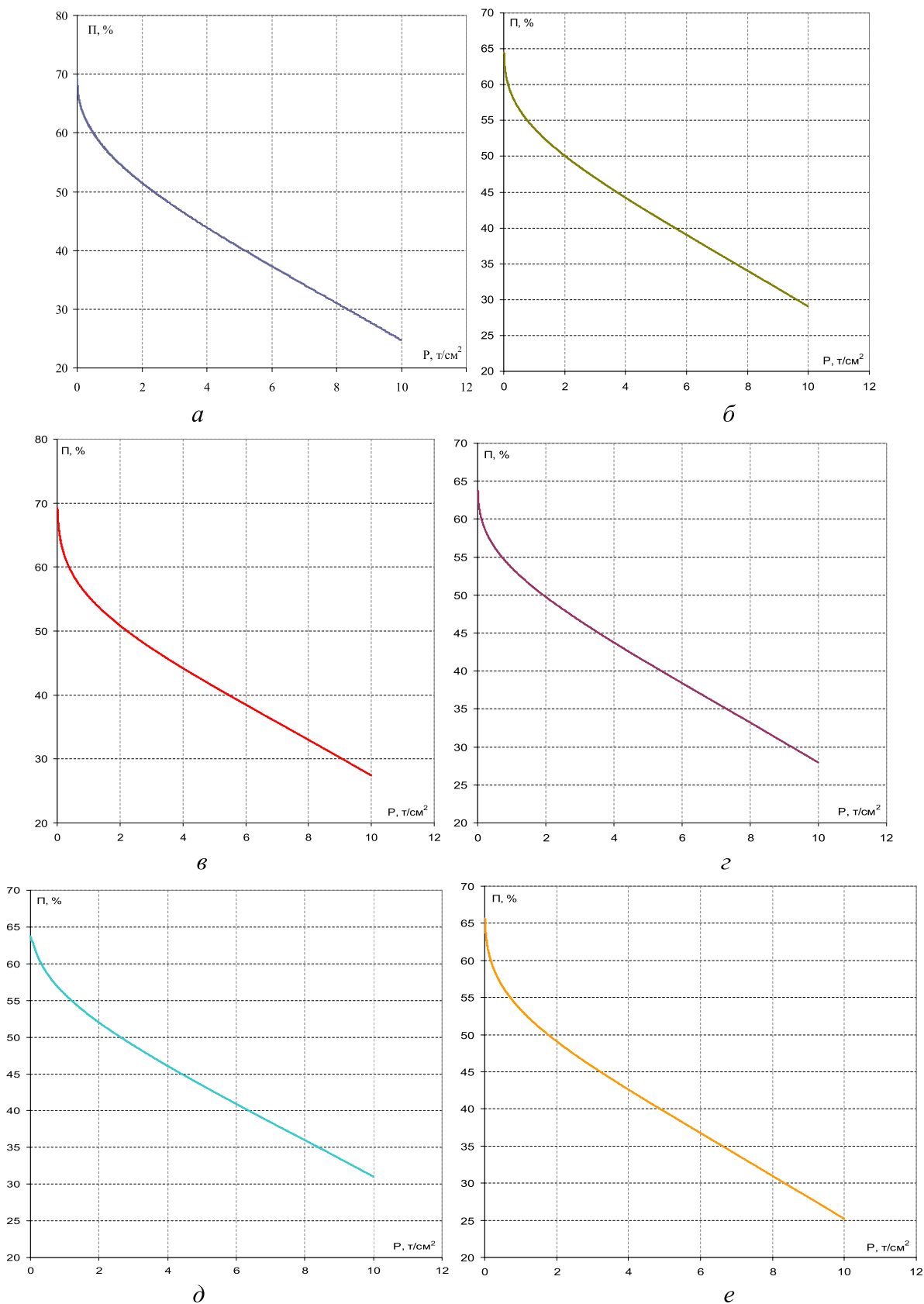
Рис. 3. Зависимости пористости от давления прессования для смесей а – [25% Co+25% Fe+50% Cu] +30% Ni; б – [25% Co+25% Fe+50% Cu] +30% Ni, 3 мин МППП; в – [25% Co+25% Fe+50% Cu] +30% Ni, 6 мин МППП; г – [[25% Co+25% Fe+50% Cu] +30% Ni]+5,3%WC, 3 мин МППП; д – [[25% Co+25% Fe+50% Cu] +30% Ni]+1,3% ZrO 2 3 мин МППП; е – [[25% Co+25% Fe+50% Cu] +30% Ni]+5,3% WC, 6 мин МППП
