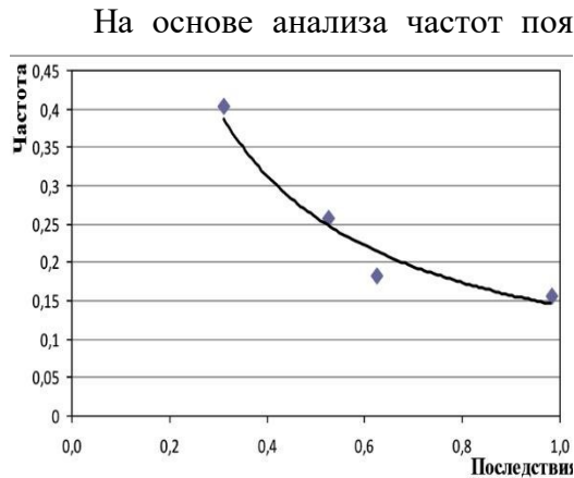
Рис. 3. Взаимосвязь между частотой неправильно принятых решений и обобщённым показателем последствий (кривая постоянного риска)
