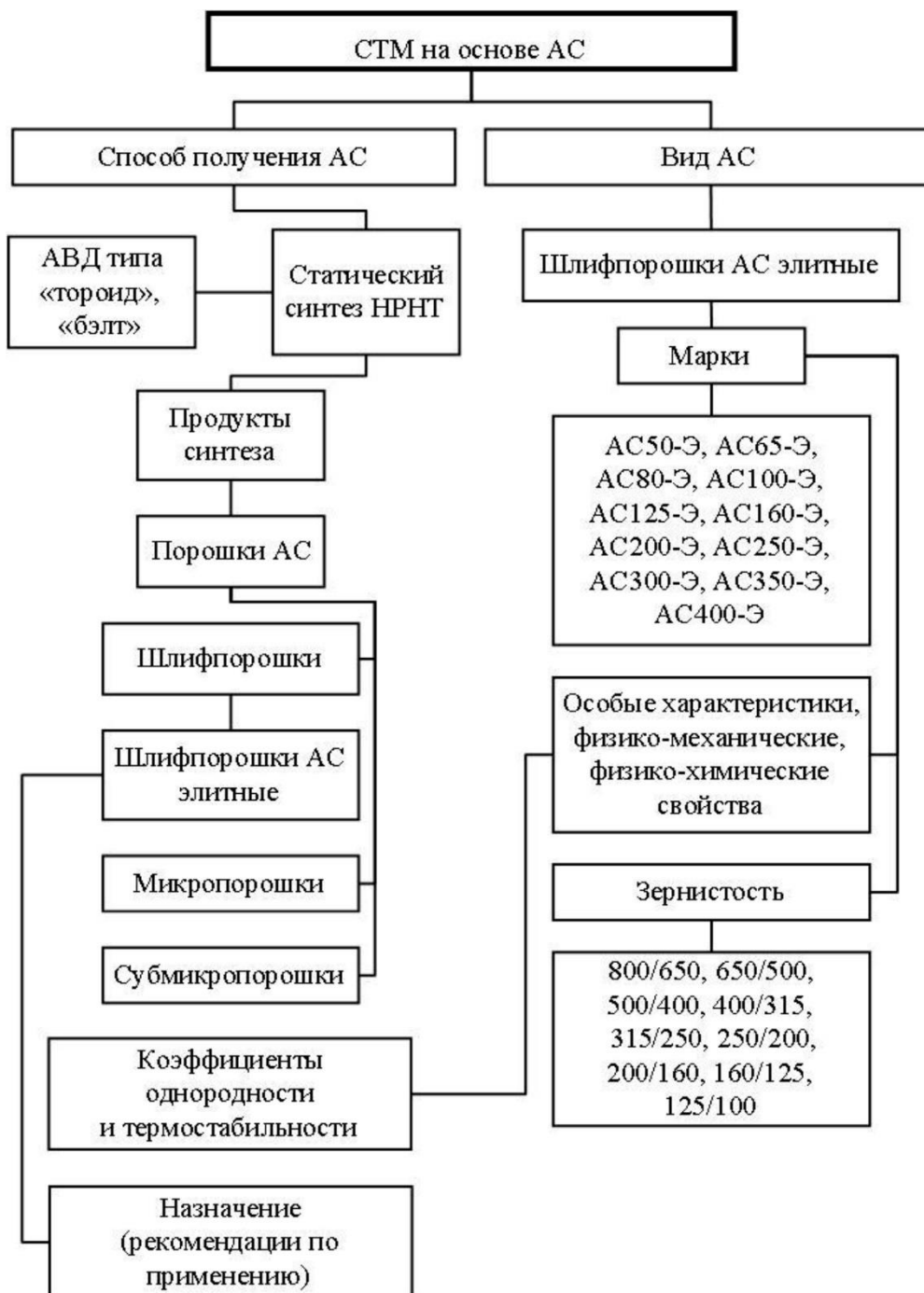
Подсистема онтологии: «Шлифпорошки из синтетических алмазов элитных для бурового и камнеобрабатывающего инструмента»
