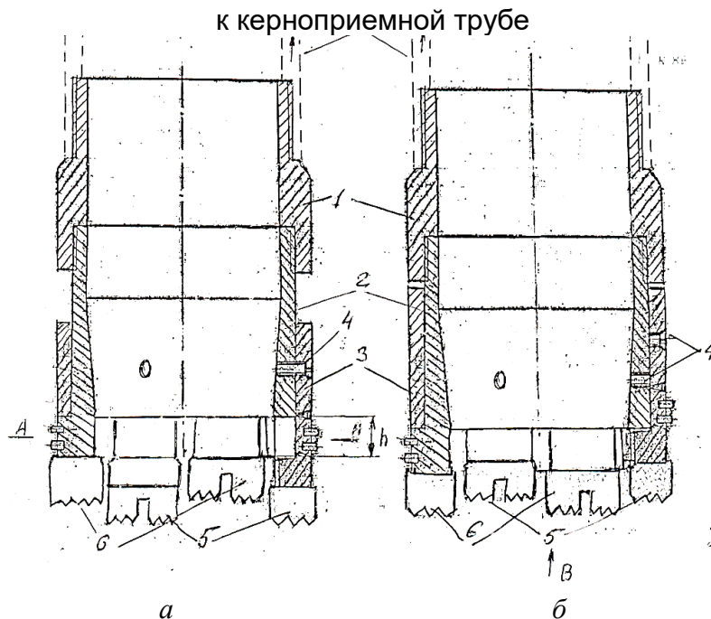
Рис 1. Принципиальная схема буровой коронки повышенной стойкости: а – положение деталей при разрушении забоя резами 5; б – положение деталей при разрушении забоя резами 6
