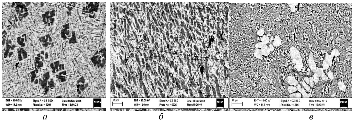
Рис. 6. Мікроструктура на гребнях валиків металу, наплавленого ПД Х10Р3Г2С без (а) та з використанням вертикальної (б) та горизонтальної (в) вібрації амплітудою 300 мкм
