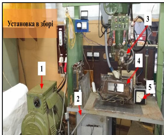
Рис. 2. Установка для наплавлення за додаткової вібрації деталі: 1 – джерело живлення генератор ПСО 500; 2 – силовий контактор; 3 – подаючий механізм ПД підвісної головки АБС; 4 – вібраційний стіл; 5 – автотрансформатор.
