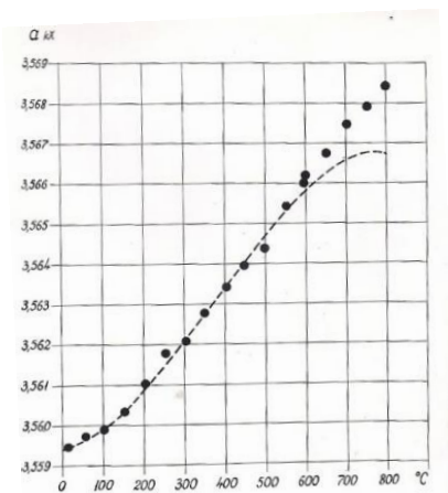
Рис. 4. Зависимость периода решетки синтетического алмаза от температуры
