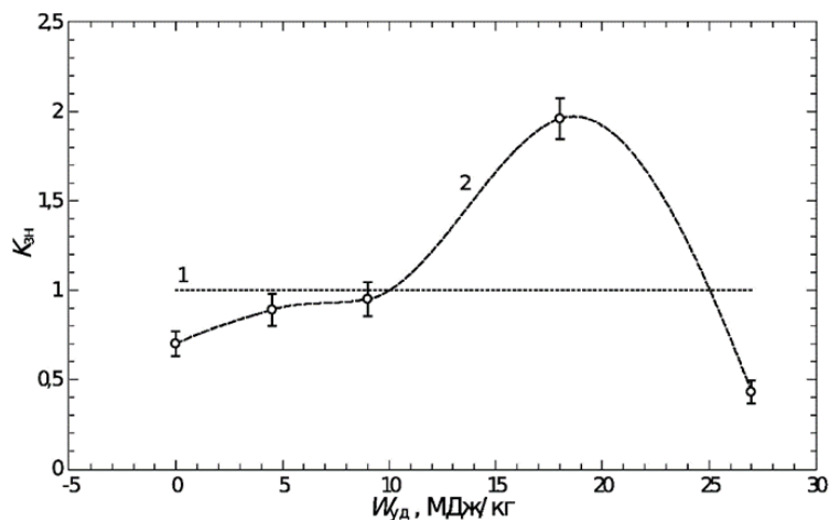
Рис. 1. Относительная износостойкость K_{зн} твердых сплавов марки ВК8 (1) и синтезированных из шихты после ВЭР (2)
