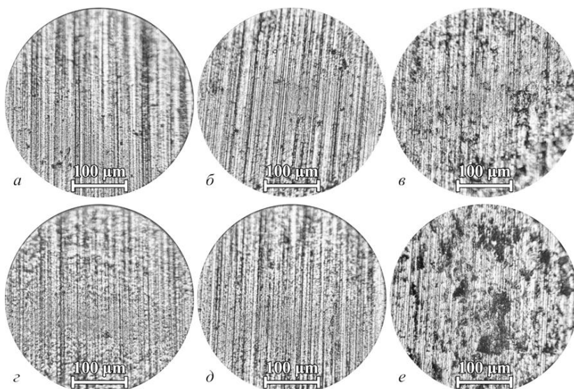
Рис. 2. Микроструктура после абразивного износа образцов сплава ВК8 (а), спеченных из исходной шихты (б) и после ВЭР обработки с удельной энергией 4,5 (в), 9 (г), 18 (д) и 27 МДж/кг (е) (оптический микроскоп, \times 40 )
