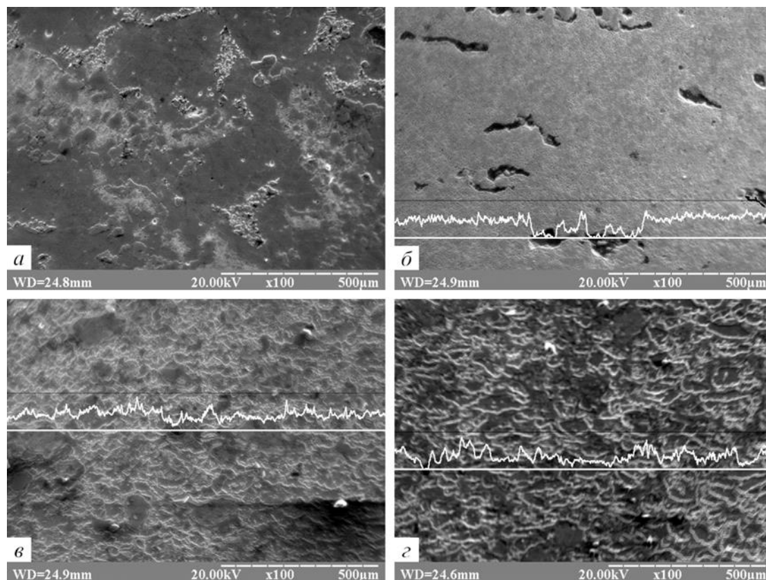
Рис. 3. Микроструктура и относительная электропроводность образцов, спеченных из исходной шихты ( а ), после ВЭР обработки с удельной энергией 4,5 ( б ), 9 ( в ), 18 МДж/кг ( з ) (электронный микроскоп, \times 100 )
