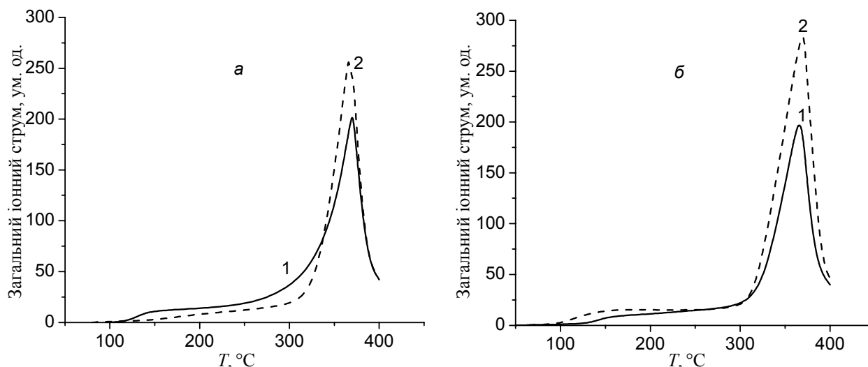
Рисунок. Температурна залежність загального йонного струму виділення летких продуктів термодеструкції зразка 1 (а) та зразка 3 (б) до (крива 1) і після (крива 2) дії культури дріжджів-аскоміцетів Y. Lipolytica
