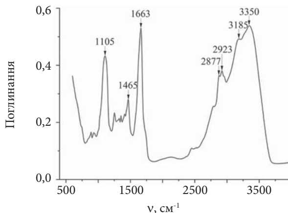
Рис. 1. ІЧ спектр ГО-1
