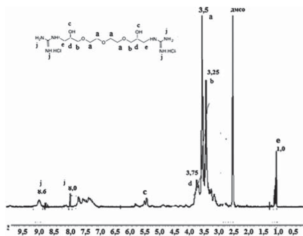
Рис. 2. 1 Н ЯМР спектр ГО-1
