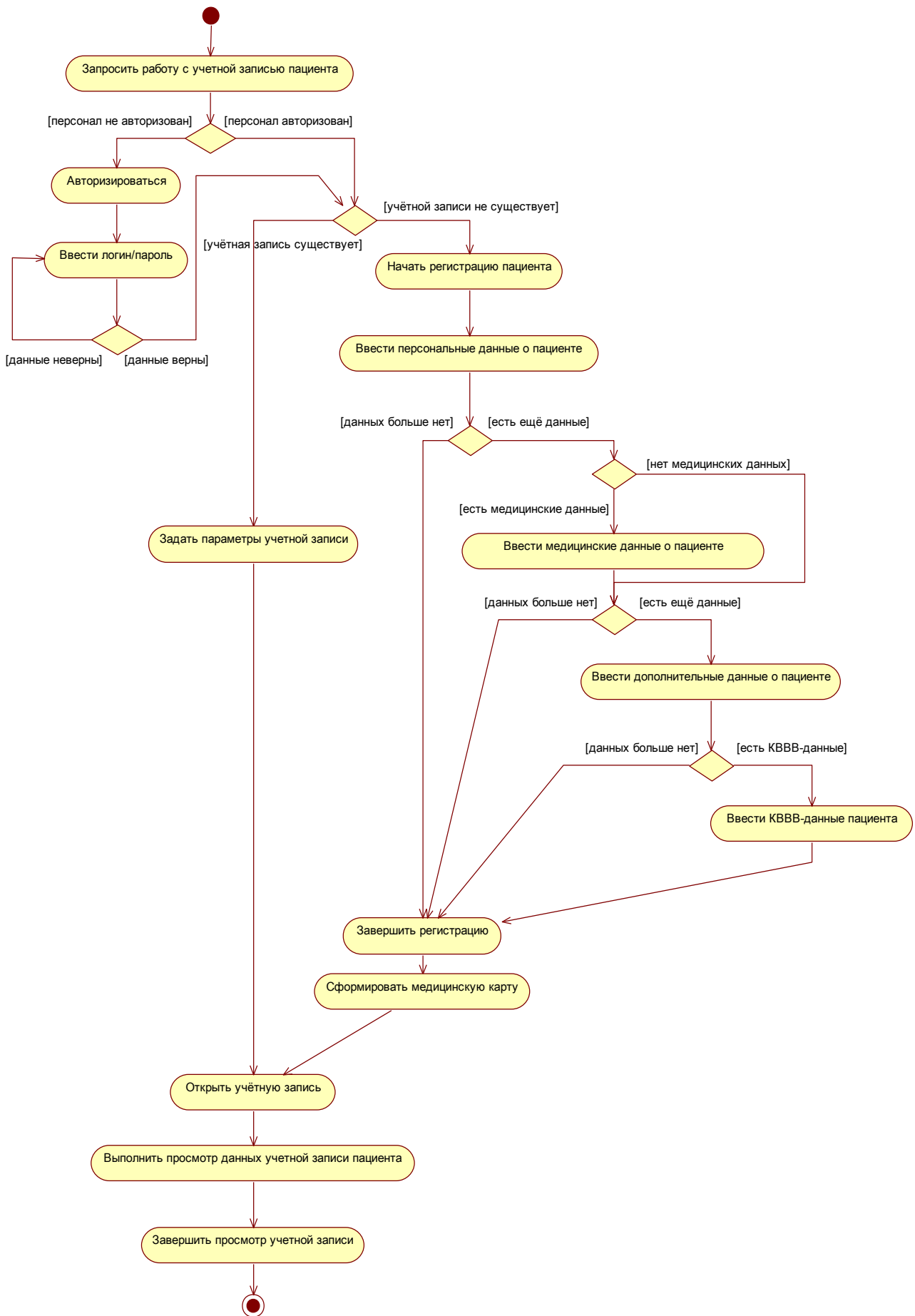
Рис. 2. Диаграмма деятельности (activity diagram) для процесса «Просмотр/создание учетной записи пациента»
