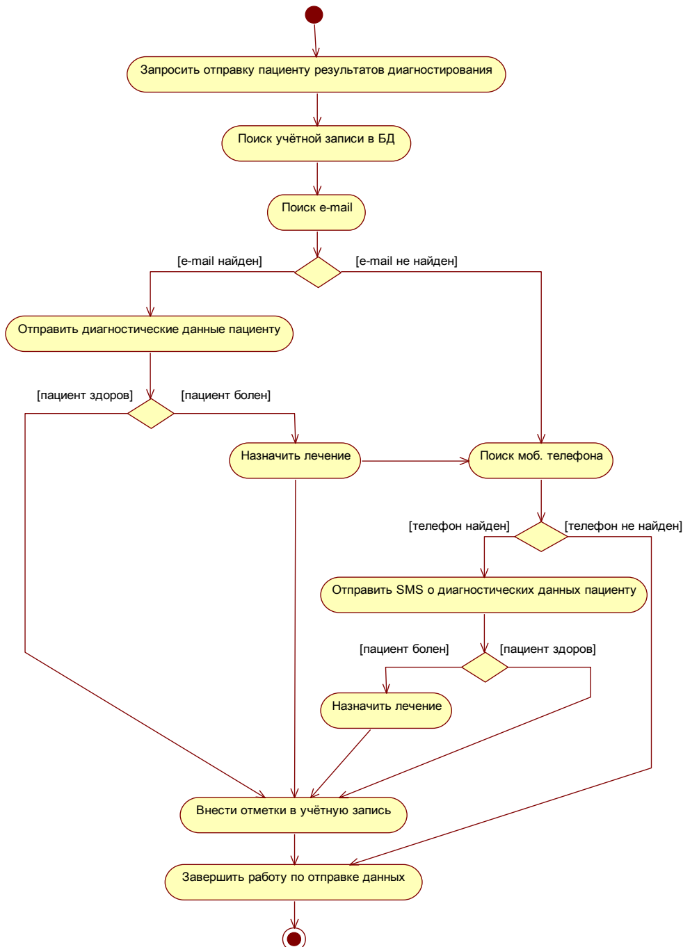
Рис. 4. Диаграмма деятельности для процесса «Отправка пациенту результатов диагностирования»
