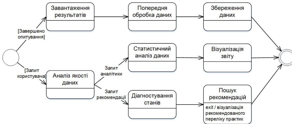
Рис. 4. Діаграма станів загального процесу роботи СППР
