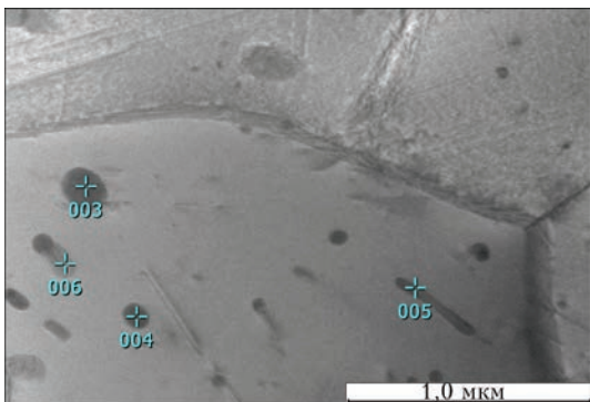
Рис. 8. Микроструктура сплава Э110М в исходном состоянии
