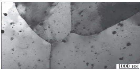
Рис. 8. Микроструктура сплава Э110М в исходном состоянии
