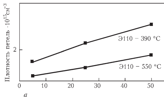
Рис. 11. Эволюция петель a -типа в сплаве Э110: a – плотность; б – размер
