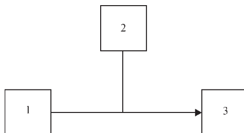
Рис. 4. Схема для контроля параметров НЧ каналов: 1 – источник постоянного тока Б5-43; 2 – измеритель напряжения Щ 4300; 3 – система ЕМА
