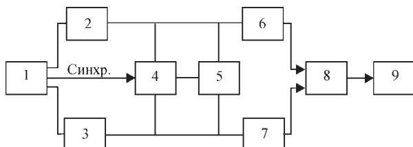
Рис. 3. Схема для контроля погрешности при измерении РВИ: 1 – генератор импульсов двухканальный Г5-56; 2, 3 – генератор сигналов специальной формы Г6-28; 4 – осциллограф двухканальный С1-85; 5 – частотомер Ч3-33; 6, 7 – переходный конденсатор емкостью 5 мкФ; 8 – промежуточный усилитель; 9 – система ЕМА
