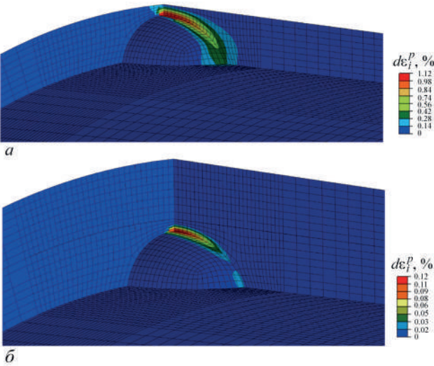
Рис. 7. Розподіл приросту інтенсивності пластичних деформацій d\varepsilon_i^p ділянки трубопроводу з дефектом: а – без підсилюючої конструкції d\varepsilon_i^p = 1,12\% ; б – з підсилюючою конструкцією d\varepsilon_i^p = 0,12\% (на порядок нижче)
