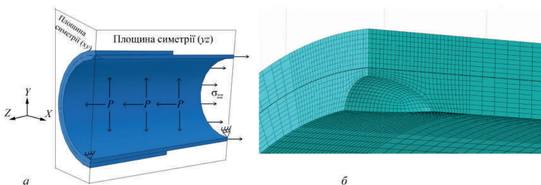
Рис. 5. Скінченно-елементна модель прямолинійної ділянки трубопроводу з дефектом стоншення стінки та підсилюючою конструкцією: а – схема моделі; б – сітка скінчених елементів в зоні дефекту
