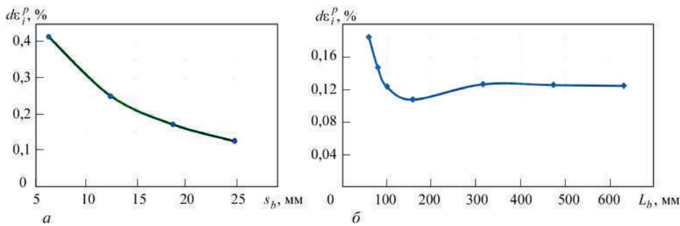
Рис. 9. Залежність максимальних значень приросту інтенсивності пластичних деформацій d\epsilon_p^p в зоні дефекту ЕКЗ трубопроводу ( D = 630 мм, s = 25 мм) від геометричних параметрів підсилюючої конструкції: а – товщини s_b ; б – напівдовжини L_b
