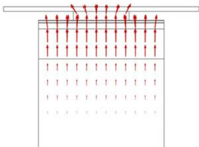
Рис.4. Розподіл ліній густини теплового потоку в біологічній тканині, на поверхні якої знаходиться термоелектричний тепломір з тепловою ізоляцією
