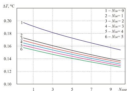
Рис.12. Залежність перепаду температур на термоелектричному тепломірі від товщини теплової ізоляції на тепломірі (кількості зовнішніх шарів бинту N_{\text{зовн}} ) при різній товщині теплової ізоляції між біологічною тканиною та тепломіром (кількості внутрішніх шарів бинту N_{\text{вн}} ) для випадку, коли зовнішня тепла ізоляція не виходить за межі верхньої грані тепломіра
