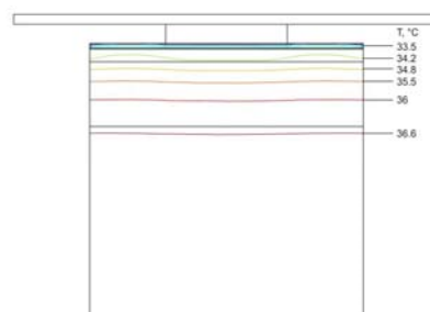
Рис.7. Ізотермічні поверхні в біологічній тканині, на поверхні якої знаходиться термоелектричний тепломір з тепловою ізоляцією
