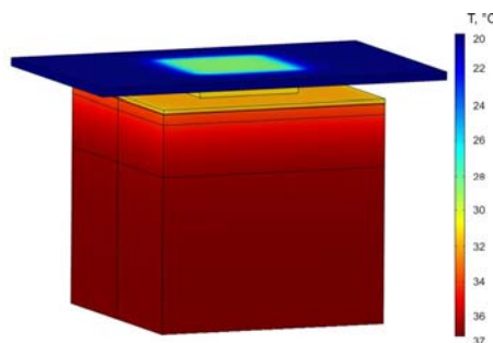
Рис.3. Розподіл температури в біологічній тканині, на поверхні якої знаходиться термоелектричний тепломір з тепловою ізоляцією
