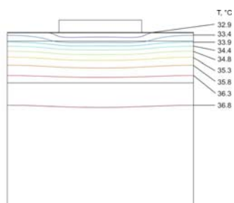
Рис.6. Ізотермічні поверхні в біологічній тканині, на поверхні якої знаходиться термоелектричний тепломір без теплової ізоляції
