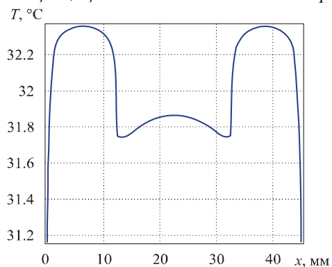
Рис.10. Розподіл температури на поверхні біологічної тканини, на якій знаходиться термоелектричний тепломір з тепловою ізоляцією
