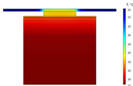
Рис.5. Розподіл температури в розрізі біологічної тканини, на поверхні якої знаходиться термоелектричний тепломір з тепловою ізоляцією
