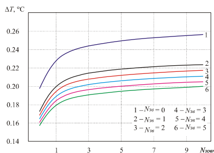
Рис.13. Залежність перепаду температур на термоелектричному тепломірі від товщини теплової ізоляції на тепломірі (кількості зовнішніх шарів бинту N_{\text{зовн}} ) при різній товщині теплової ізоляції між біологічною тканиною та тепломіром (кількості внутрішніх шарів бинту N_{\text{вн}} ) згідно фізичної моделі, коли зовнішня тепла ізоляція виходить за межі тепломіра
