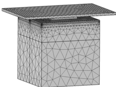
Рис.2. Сітка методу скінченних елементів
