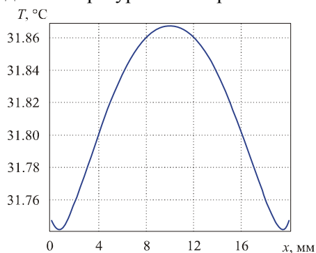
Рис.8. Розподіл температури на нижній поверхні термоелектричного тепломіра з тепловою ізоляцією, що виходить за межі тепломіра
