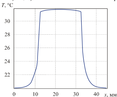
Рис.11. Розподіл температури на поверхні теплової ізоляції, що знаходиться на термоелектричному тепломірі
