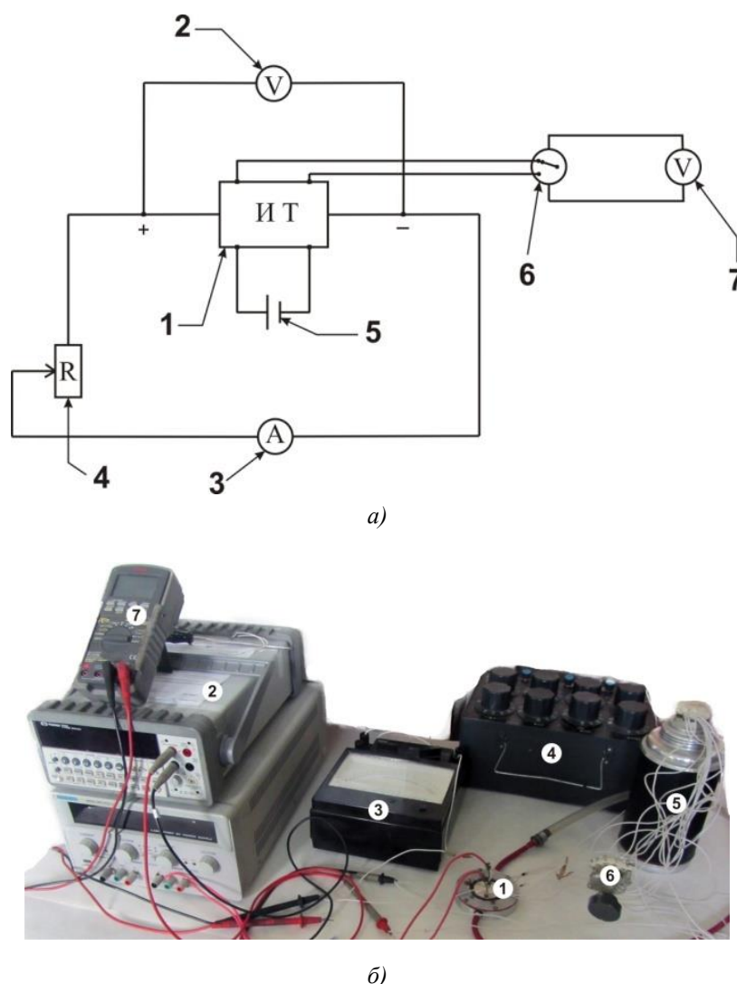
Рис. 4. Схема (а) і зовнішній вигляд(б) експериментального стенду для дослідження макетних зразків ДС :
