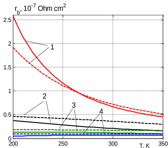
Рис. 4. Температурні залежності питомого опору границі r_b для контактів нікелю з ТЕМ Bi_2Te_{2.7}Se_{0.3} n-типу провідності (суцільні лінії) та Bi_{0.5}Sb_{1.5}Te_3 p-типу (пунктирні лінії), розраховані для різних концентрацій легуючих домішок N_d в приконтактному шарі ТЕМ: 1 – оптимальна концентрація в ТЕМ, 2 – N_d = 10^{26} \text{ м}^{-3} , 3 – N_d = 1.5 \cdot 10^{26} \text{ м}^{-3} , 4 – N_d = 2 \cdot 10^{26} \text{ м}^{-3} .
