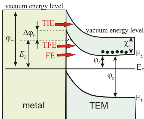
Рис.2. Діаграма енергетичних зон контакту металу з термоелектричним матеріалом n-типу провідності. Механізми проходження електронів через потенціальний бар'єр:
