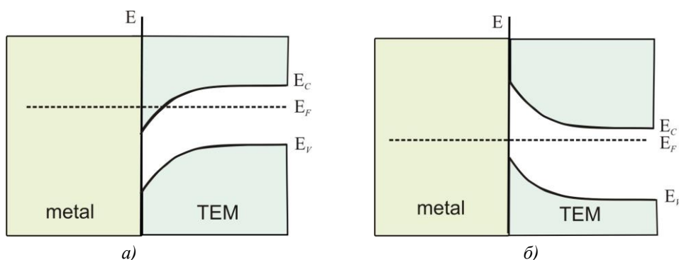
Рис. 1. Викривлення енергетичних зон напівпровідника в зоні контакту з металом.
