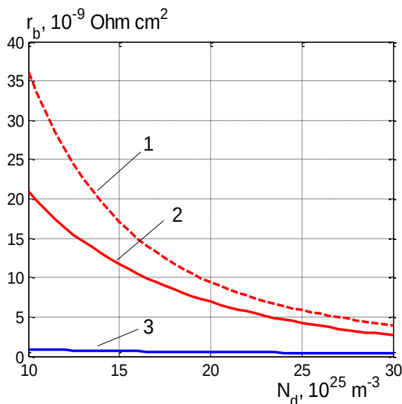
Рис.6. Залежності питомого опору границі r_b від концентрації домішок N_d в приконтактному з нікелем шарі ТЕМ \text{Bi}_{0.5}\text{Sb}_{1.5}\text{Te}_3 p-типу (1) та \text{Bi}_2\text{Te}_{2.7}\text{Se}_{0.3} n-типу провідності (2) за умови T=300 \text{ К} . 3 – залежності мінімального питомого опору r_{b \min}(N_d) практично співпадають для ТЕМ p- і n-типу провідності.
