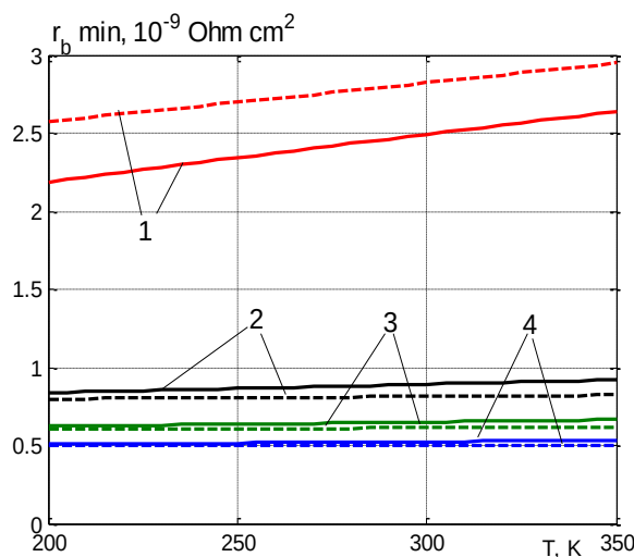
Рис. 5. Температурні залежності мінімального питомого опору границі r_{b \min} для контактів нікелю з ТЕМ Bi_2Te_{2.7}Se_{0.3} n-типу провідності (суцільні лінії) та Bi_{0.5}Sb_{1.5}Te_3 p-типу (пунктирні лінії), розраховані для
