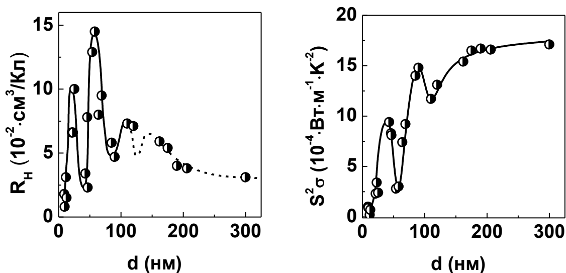
Рис. 1. Залежності електропровідності \sigma (а), коефіцієнта Зеебека S (б), коефіцієнта Холла R_H (в) і термоелектричної потужності P = S^2 \sigma (г) при кімнатній температурі в ід товщини d плівок Bi_{0.98}Sb_{0.02} , виготовлених методом термічного випаровування у вакуумі на підкладки зі слюди. На рис. 1,а) показана пунктиром теоретична залежність \Delta(d) , одержана з використанням теорії Фукса - Зондгеймера.
