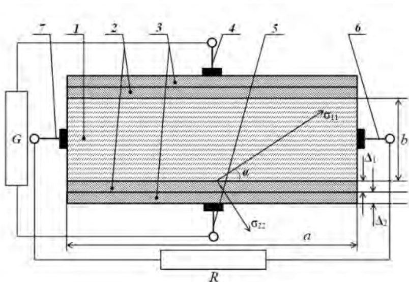
Рис. 5. Схематичне зображення конструкції АЕГ 1 – Пластина з анізотропного електропровідного матеріалу; 2 – електроізоляційні шари; 3 – електропровідні шари; 4, 5 – входні; 6, 7 – вихідні електровиводи.
