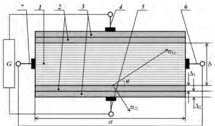
Рис. 6. Схематичне зображення конструкції АЕН 1 – Пластина з анізотропного електропровідного матеріалу; 2 – електроізоляційні шари; 3 – електропровідні шари; 4, 5 – вхідні; 6, 7 – вихідні електровиводи.
