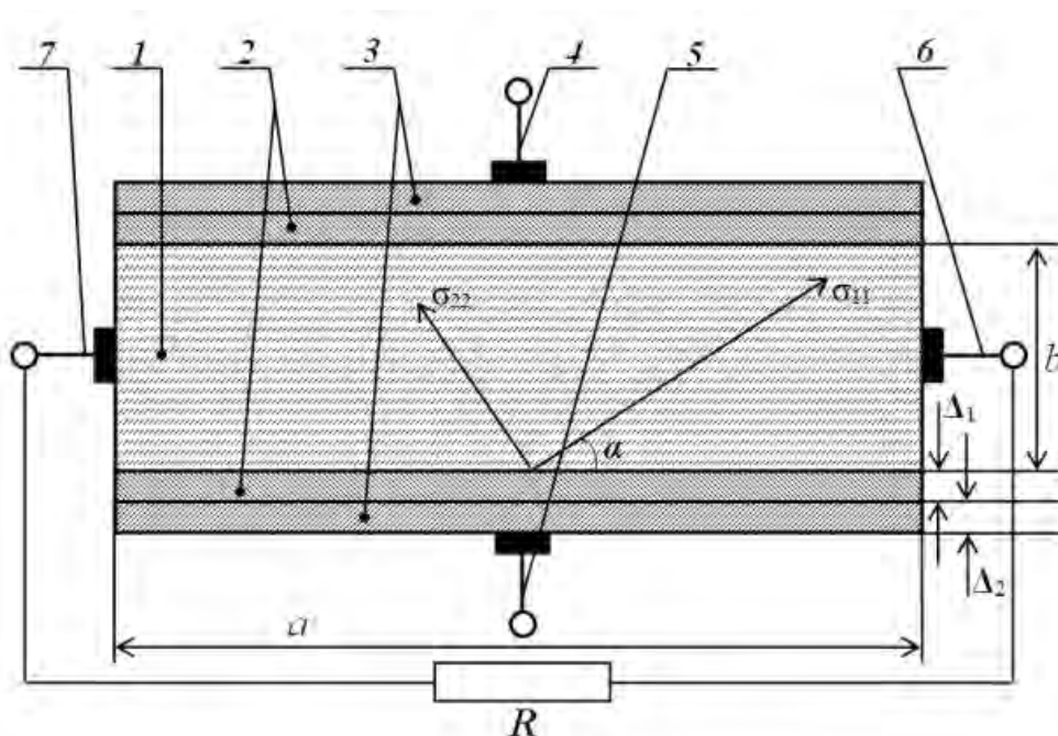
Рис. 1. Схематичне зображення конструкції анізотропного трансформатора 1 – Пластина з анізотропного електропровідного матеріалу; 2 – електроізоляційні шари; 3 – електропровідні шари; 4, 5 – вхідні; 6, 7 – вихідні електровиводи.
