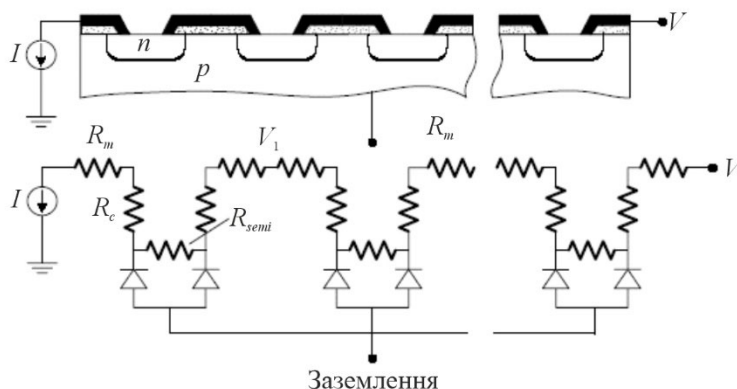
Рис. 4. Схема багатоcontactного двоклемного методу [10].
