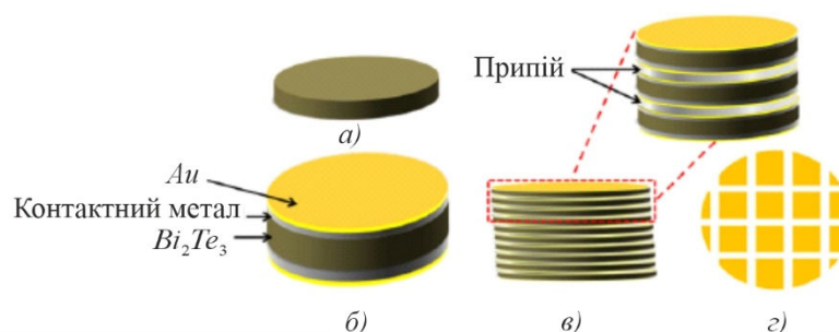
Рис. 14. Послідовні стадії процесу виготовлення зразків [11]: а) – одинична пластина після притирання; б) – пластина після травлення і осадження контактного шару; в) – готова пачка з 10 пластин після спаювання; г) – пачка пластин, розрізана на кубики.
