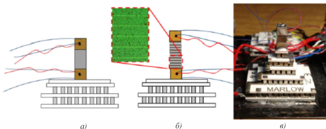
Рис. 13. Спосіб вимірювання контактного опору за добротністю [11]: а) – контрольний зразок; б) – пачкоподібна структура; в) – загальний вигляд вимірювального стенду.
