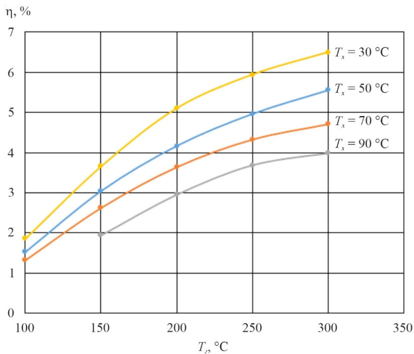
Рис. 6. Залежність ККД \eta термоелектричного модуля типу Altec-1061 від температур гарячої T_z та холодної T_x сторін модуля.
