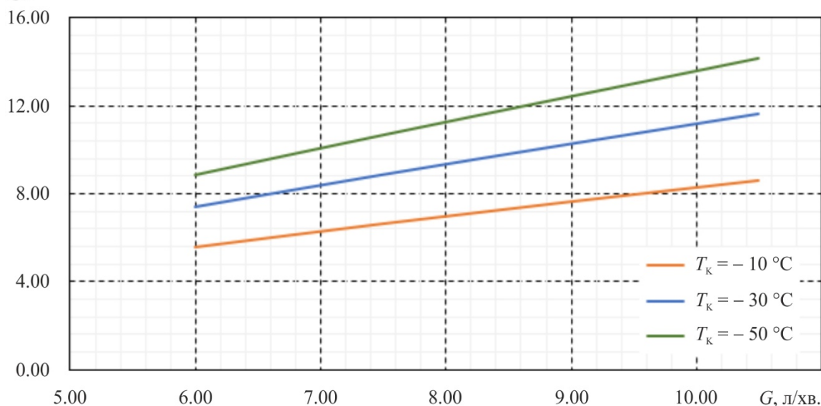
Рис. 7. Залежності теплової потужності Q_0 , яку необхідно відвести від робочої камери, від витрати видихуваного повітря G для різних значень температури робочої камери T_k (при температурі видихуваного повітря 33.5^\circ\text{C} та його відносній вологості 90 %).
