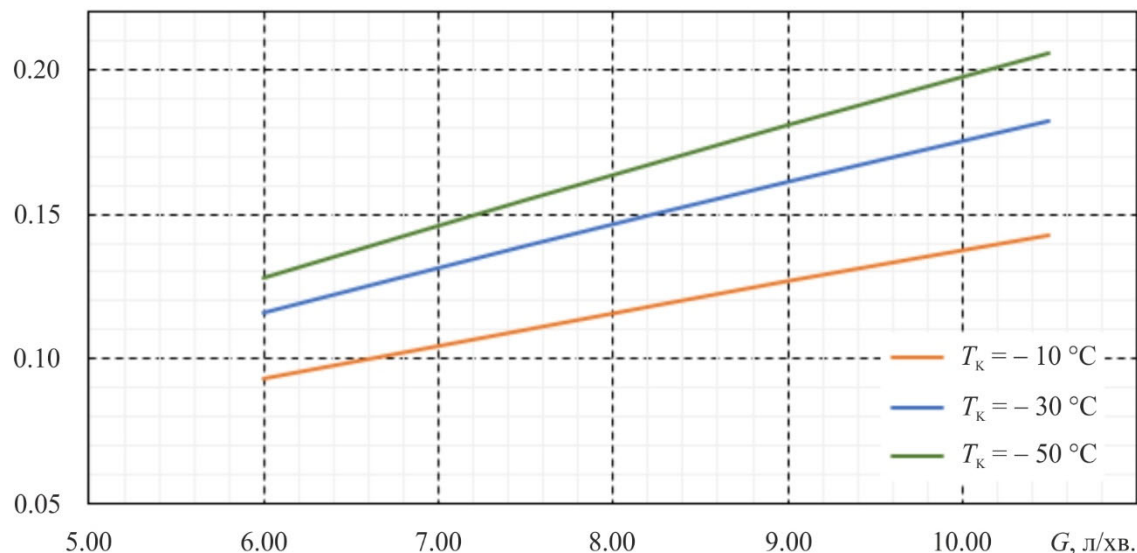
Рис. 6. Залежності швидкості збирання конденсату V_k від витрати видихуваного повітря G для різних значень температури робочої камери T_k (при температурі видихуваного повітря 33.5^\circ\text{C} та його відносній вологості 90%).
