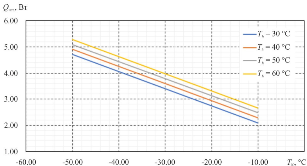
Рис. 7. Залежності натікань тепла з оточуючого середовища до робочої камери Q_{\text{нат}} від температури робочої камери T_K для різних значень температури гарячої сторони термоелектричного модуля (температура додаткової камери -0\text{ }^{\circ}\text{C} ).
