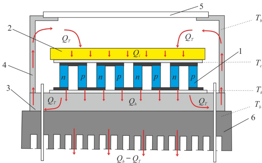
Рис. 7. Фізична модель оптико-електронного пристрою з ТЕО в металевому корпусі [16]. 1 – ТЕО, 2 – оптико-електронний елемент, 3 – цокольна пластина корпусу, 4 – кришка корпусу, 5 – вікно, 6 – основа теплообмінника.
