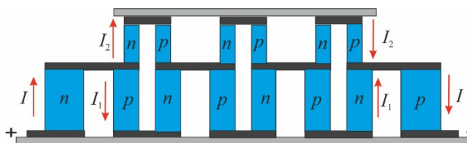
Рис. 4. Модель ТЕО з паралельним живленням каскадів.
