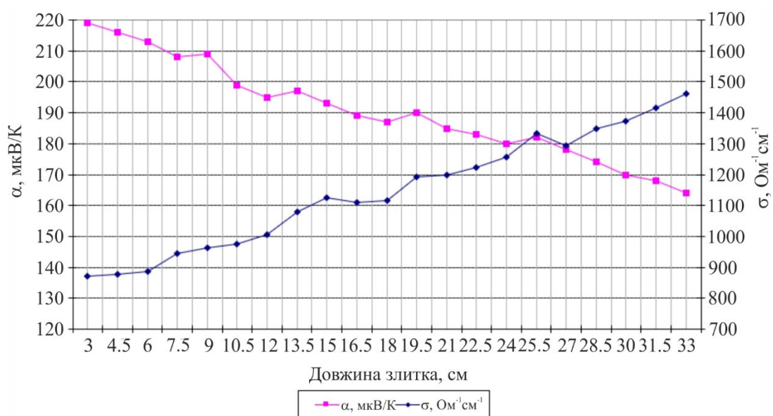
Рис. 4. Термоелектричні параметри, де h = 1.5 d .
