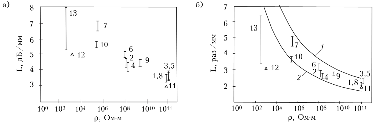
Рис. 1. Значения коэффициента поглощения L ( a – в дБ/мм, b – в раз/мм) и соответствующее ему объемное удельное электрическое сопротивление для материалов, приведенных в таблице (цифры соответствуют порядковому номеру материала)
