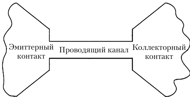
Рис. 1. Иллюстрация к описанию квантового провода
