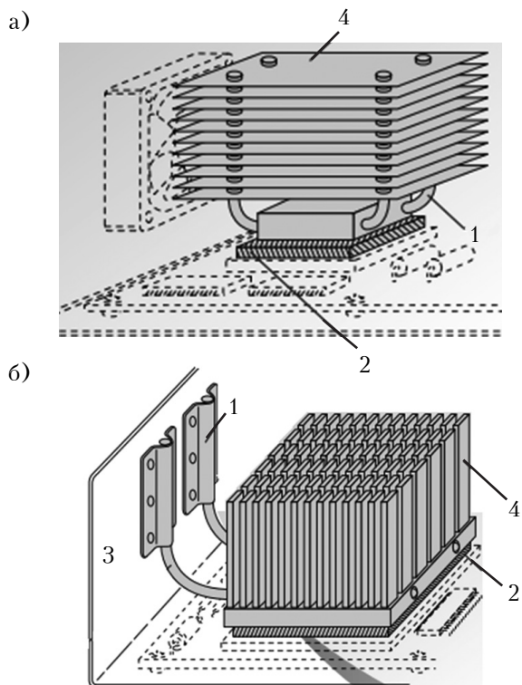
Рис. 4. Основные схемные решения использования ТТ в активной (а) и пассивной (б) системах охлаждения компьютерной техники класса десктоп [8]: 1 – ТТ; 2 – тепловыделяющие элементы; 3 – корпус (плата); 4 – радиатор
