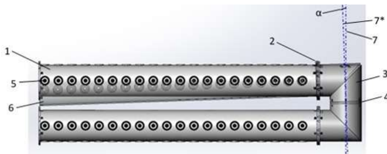
1 – труба, 2 – з'єднувальні фланці, 3 – перехідне коліно, 4 – сепаратор, 5 – кодована мішень, 6 – труба маніпулятора, нахилена у площині зображення на кут \alpha через люфт, 7 – вісь обертання шарнірного вузла маніпулятора, 7* – вісь обертання шарнірного вузла маніпулятора, відхилена на кут \alpha
