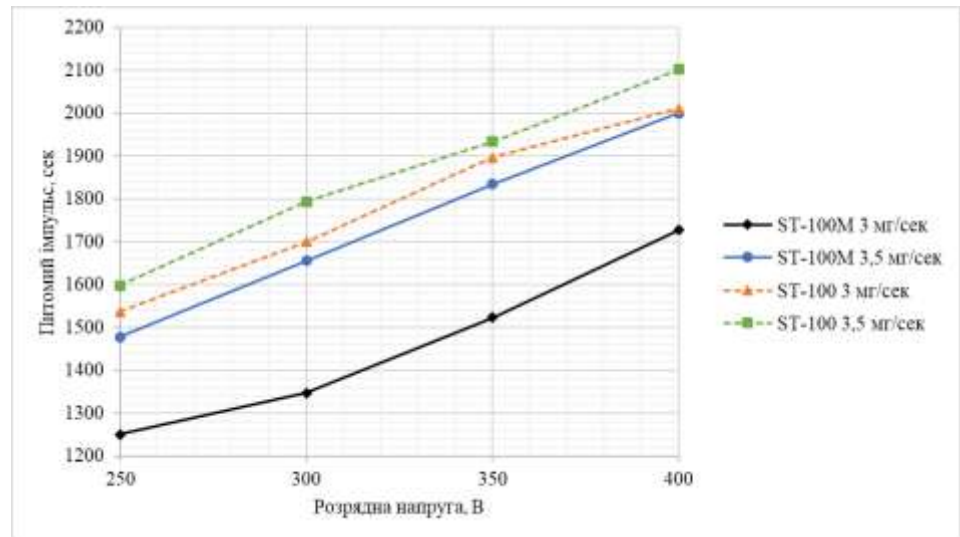
Рис. 14 – Залежність питомого імпульсу від напруги розряду при різних витратах робочого тіла (Хе)
