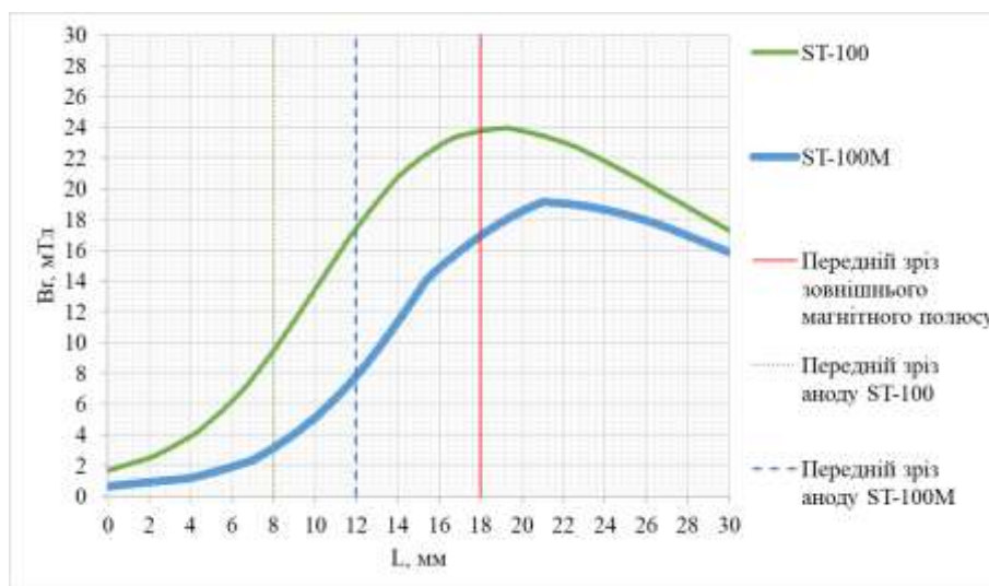
Рис. 7 – Розрахункові значення радіальної складової магнітної індукції B_r на серединній лінії розрядного каналу для ST-100 та ST-100M при однакових токах та кількості витків у котушках. L – відстань від аноду назовні
