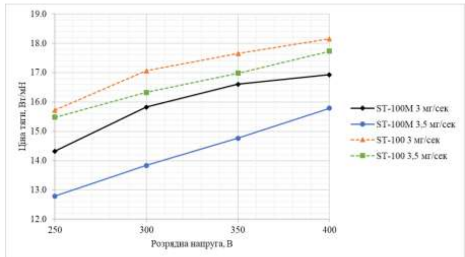
Рис. 15 – Залежність ціни тяги від напруги розряду при різних витратах робочого тіла (Хе)
