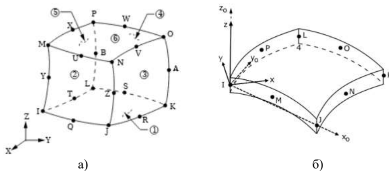
Рис. 2 – Геометрія скінченних елементів
