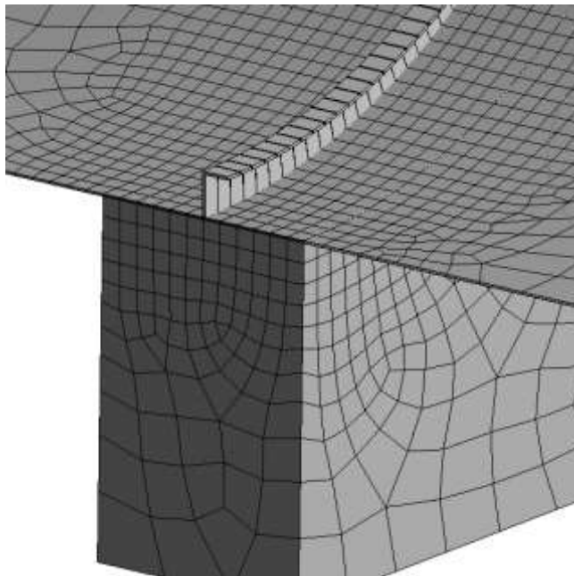
Рис. 6 – Скінченно-елементна модель контакту «ребро жорсткості–оболонка–ложемент»
