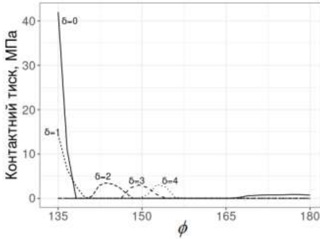
Рис. 9 – Залежність контактної тиску від кутової координати
