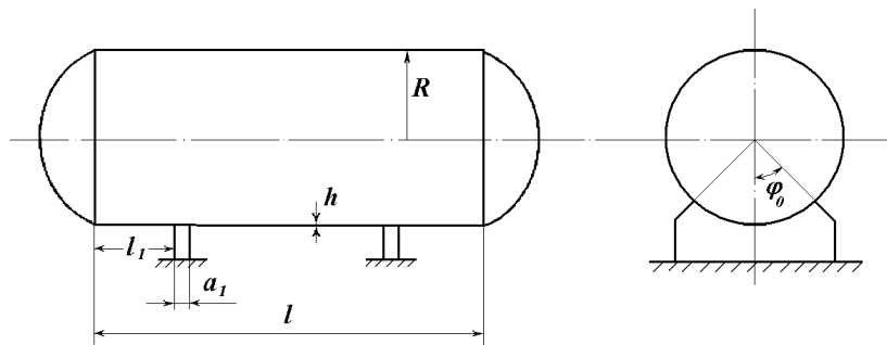
Рис. 4 – Загальна схема спирання оболонки на ложементи
