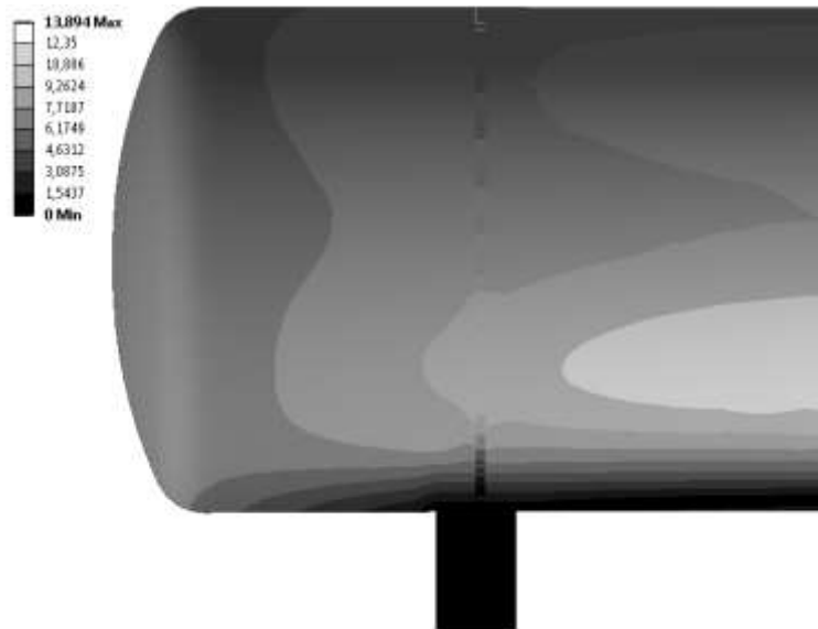
Рис. 7 – Розподіл поля деформацій в оболонці (в мм)
