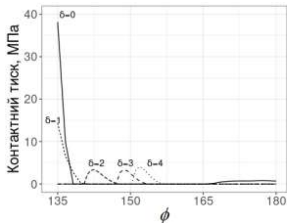
Рис. 10 – Залежність контактної тиску від кутової координати при використанні моделі Вінклера
