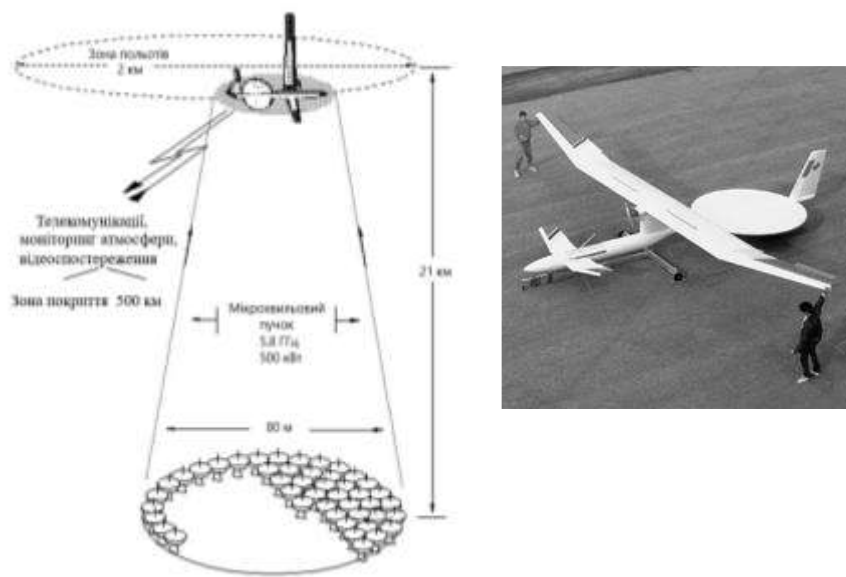
Рис. 3 – Модель і конфігурація системи SHARP [6]
