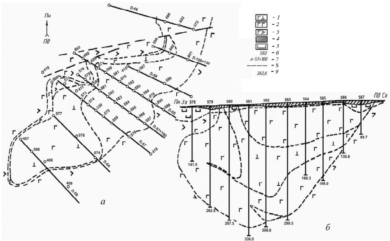
Рис. 1. Геологічна карта (а) та геологічний розріз по лінії 57+100 (б). Федорівська інтрузія. Масштаб 1:10 000: 1 – габро-перидотит рудний; 2 – габро лейкомеланократове рудне; 3 – габро-анортозит безрудний; 4 – осадові відклади; 5 – кора вивітрювання; б – свердловина та її номер; 7 – номер лінії свердловини; 8 – тектонічні порушення; 9 – глибина свердловини
