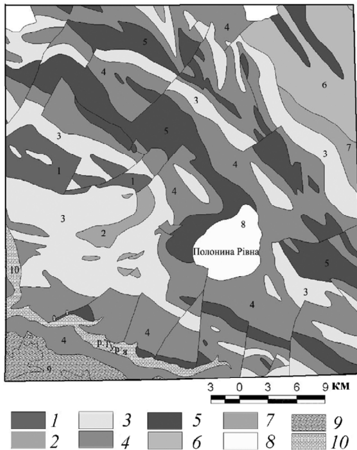
Рис. 2. Геологічна будова фрагменту території досліджень. (Світлішим тоном показані породи, більш стійкі до розмивання). Літостратиграфічні комплекси: 1 – Cr_2bz . Крейдяна система, березнинська світа, тонкоритмічний фліш із переважанням тонкоритмічних темно-сірих аргілітів, прошарками мергелей та вапняків; 2 – Cr_2sv . Крейдяна система, свидовецька світа, щільні кременисті аргіліти з прошарками пісковиків; 3 – Pg_1lt . Палеоцен, лютська світа, щільні масивні вапняковисті пісковики, з прошарками гравелітів, конгломератів та аргілітів; 4 – Pg_2 . Еоцен, тонкоритмічне перешарування пістрявих аргілітів, алевролітів та пісковиків; 5 – Pg_3^1ml_1 . Нижній олігоцен, нижньоменілітова світа, темноколірні некарбонатні аргіліти з прошарками алевролітів та пісковиків; 6 – Pg_3^2kr_1 . Середній олігоцен, нижньокросненська світа, масивні пісковики із прошарками аргілітів; 7 – Pg_3^{2-3}kr_2 . Середній та верхній олігоцен, середньокросненська світа, тонкоритмічне чергування вапняковистих алевролітів, аргілітів та пісковиків; 8 – Pg_3^3rn . Верхній олігоцен, рунська світа, масивні пісковики; 9 – N_2 . Неоген, вулканічні породи; 10 – четвертинна система, алювій, складений галечниками, валунами, гравієм, піском
