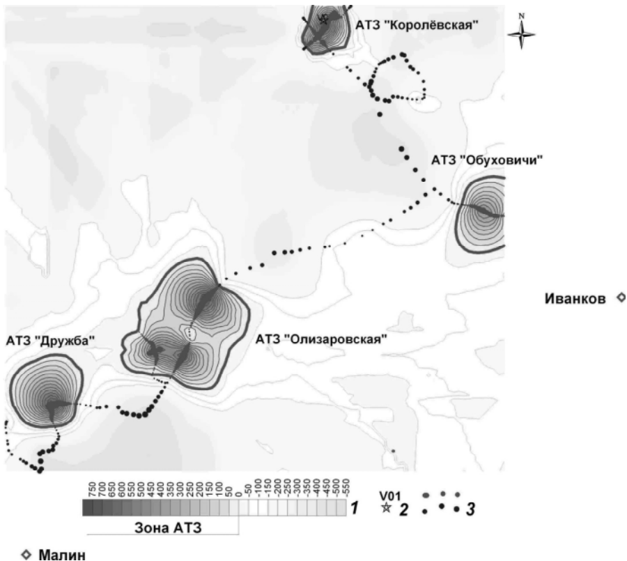
Рис. 1. Карта-схема геоелектрических аномалий типа “залежь” в районе населенных пунктов Иванков и Малин: 1 – шкала значений поля СКИП; 2 – пункт ВЭРЗ в пределах АТЗ “Королевская”; 3 – пункты съемки СКИП
