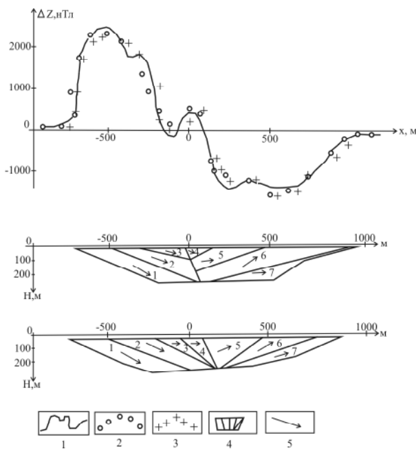
Рис. 4. Тело габброидів Кропивенського участка. Результати інтерпретації магнітної аномалії на профілі III: 1 – спостережена аномалія \Delta Z ; 2, 3 – аномалії від підібраних варіантів моделі; 4 – контури сегментів моделі (вертикальне сечення вдоволь профіля III); 5 – напрямлення векторів ефективною намагніченності сегментів
